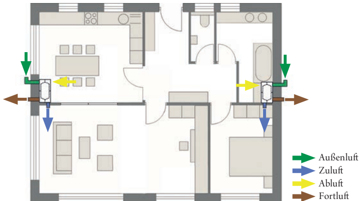
Grundriss für ein Raumverbundsystem. Zuluft in das Wohnzimmer und Abluft über Küche und Esszimmer.
