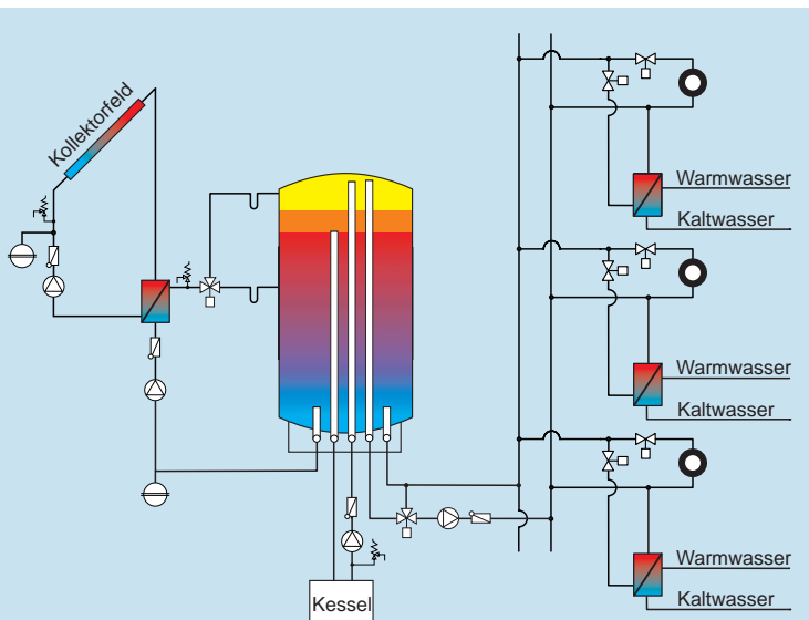
▼ Solarunterstütztes Wärmeversorgungssystem nach dem Prinzip von Zwei-Leiter-Netzen in Verbindung mit Wohnungsstationen (siehe links) als Standardversorgungssystem im Geschosswohnbau
